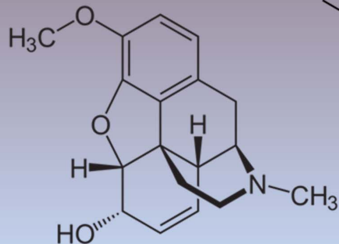
KODEIN
